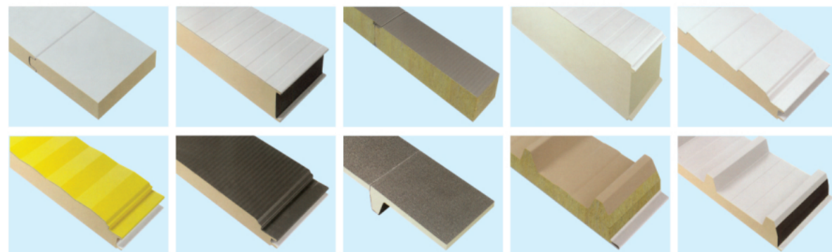
▲ 板型图 Panel profiles
